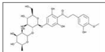
Neohesperidin CAS #: 13241-33-3
