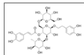
Echinacoside CAS #: 82854-37-3
