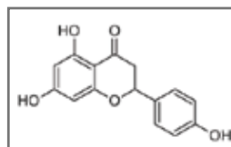
Naringenin CAS #: 480-41-1
