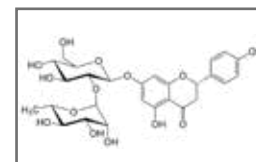
Naringin CAS #: 480-41-2
