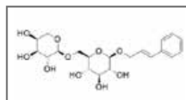
Rosavins CAS #: 84954-92-7
