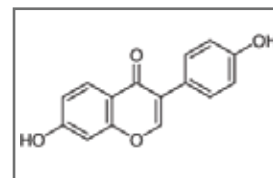
Isoflavones CAS #: 486-66-8
