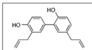
Honokiol CAS #: 35354-74-6
