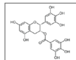
EGCG CAS #: 989-51-5
