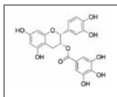
ECG CAS #: 1257-08-5
